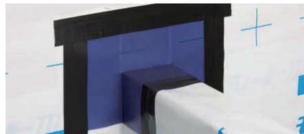
バルコニー端部 (FSK3105)
