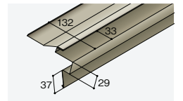
水切セットバックスターJ-29J
