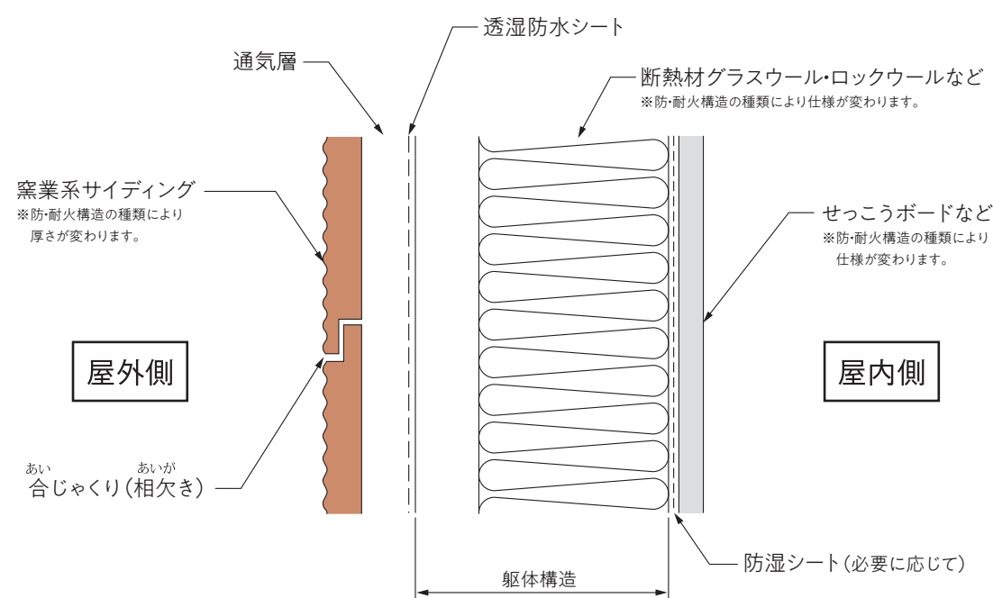
窯業系サイディングを使用した外壁部分の標準構造
