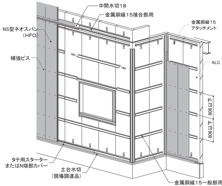
縦張り施工
