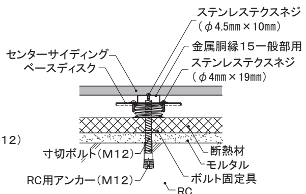
水平断面図
