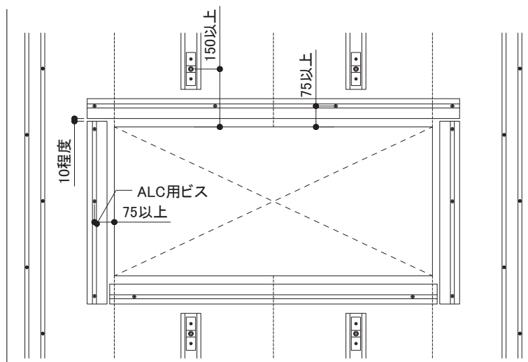
※開口部まわりは、金属胴縁15接合部用をALC用ビスで留め付けます。
