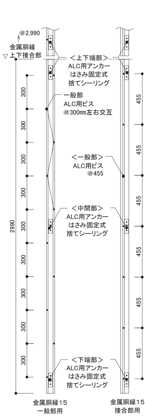
※開口部まわりは、金属胴縁15接合部用をALC用ビスで留め付けます。
