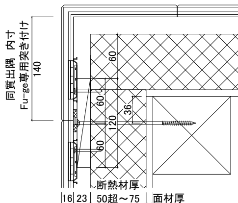
同質出隅 Fu-ge専用突き付け 内寸140mm
