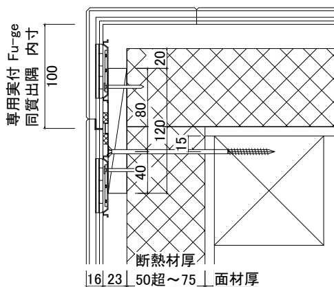
同質出隅 Fu-ge専用実付 内寸100mm
