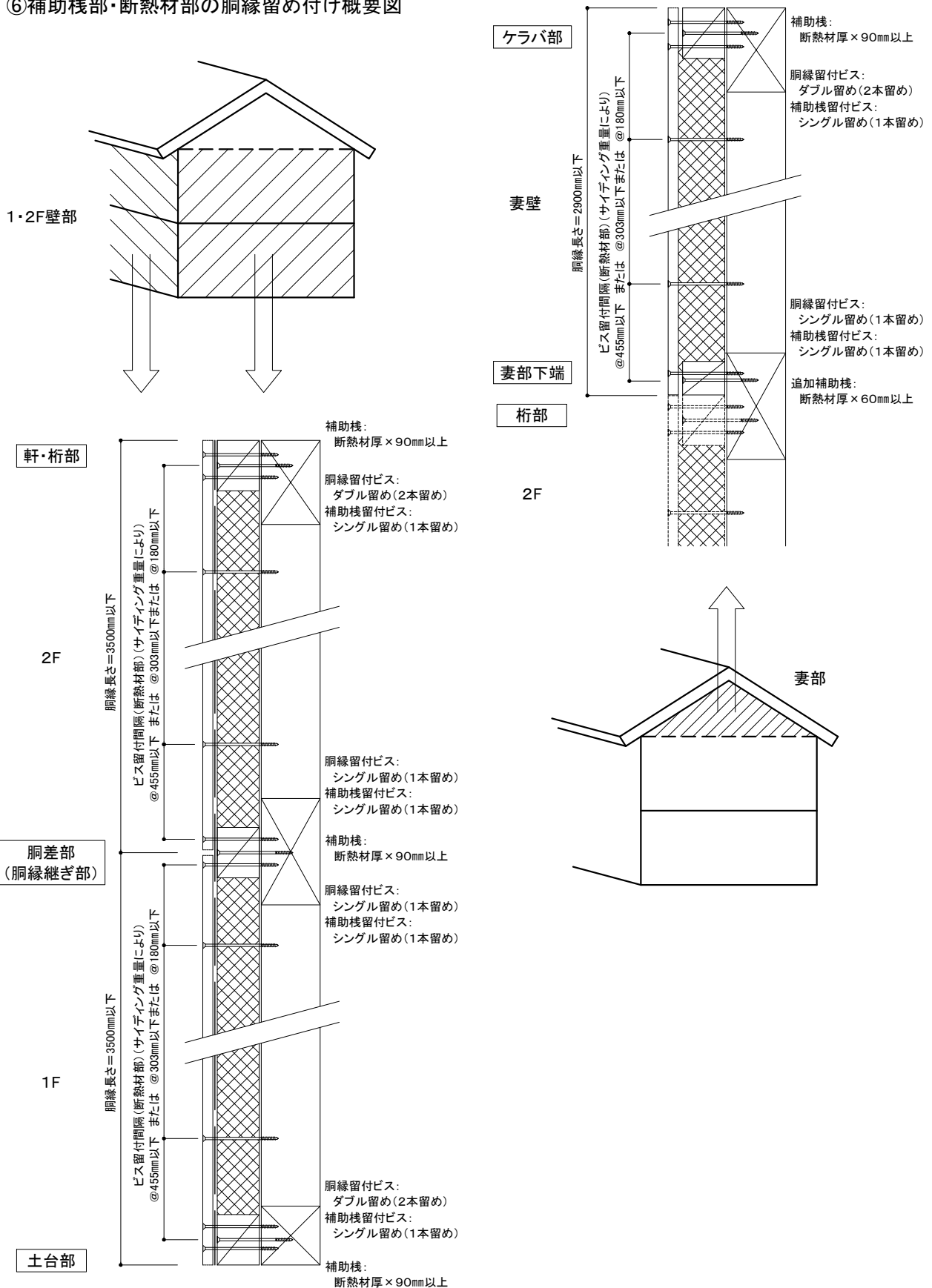
⑥補助桟部・断熱材部の胴縁留め付け概要図
