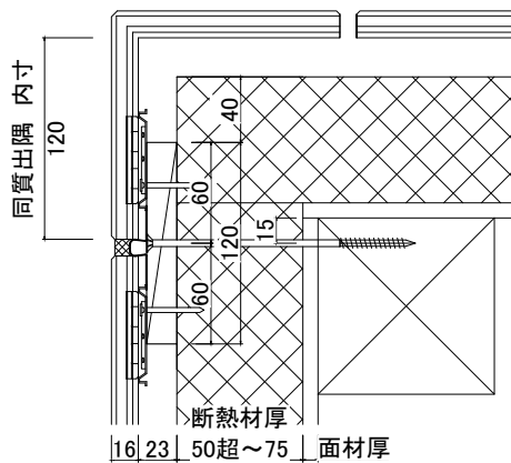
同質出隅 内寸120mm
