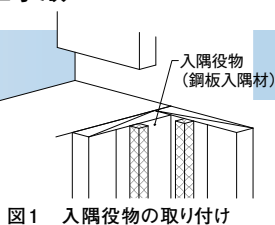
図1 入隅役物の取り付け
