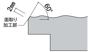
図3 面取り加工
