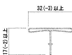
目地カバー(鋼板製)
