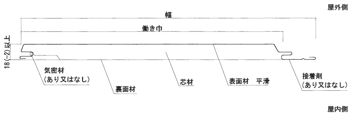
外装材断面
