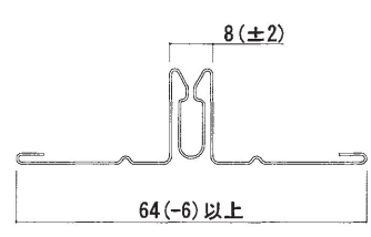
目地受け(鋼板製)
