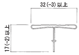
目地カバー(1ピースタイプ)
