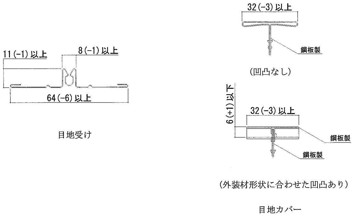
役物断面形状図 図3 構造説明図
