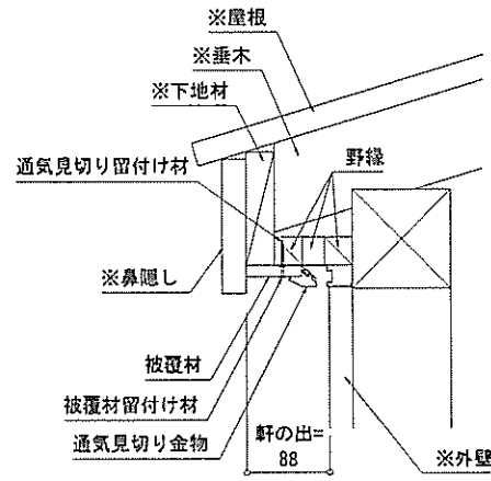
軒部詳細図（軒勝ち）
