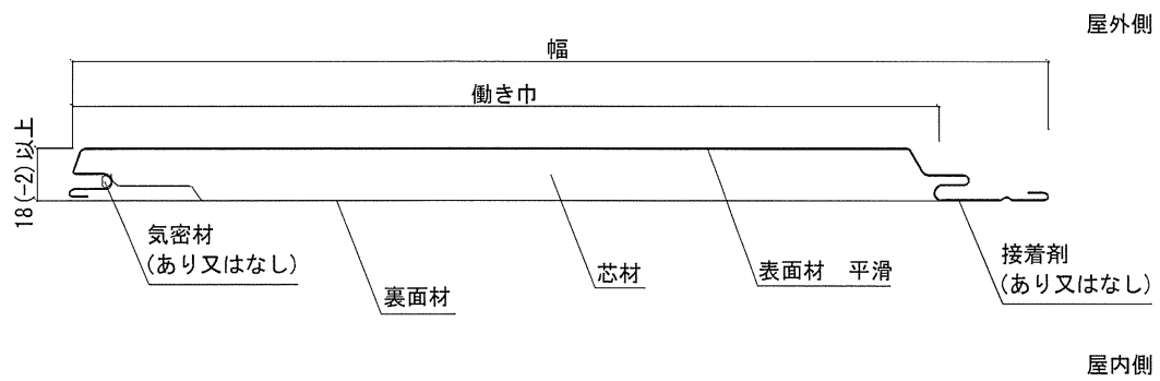
外装材断面
