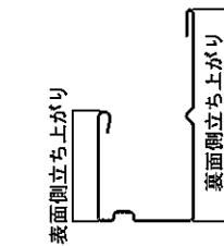
目地部材B(1ピースタイプ)
