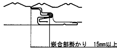
嵌合部詳細
