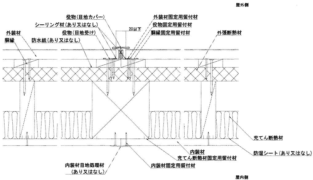
図2 構造説明図(構造用面材なし、充てん断熱材あり)
