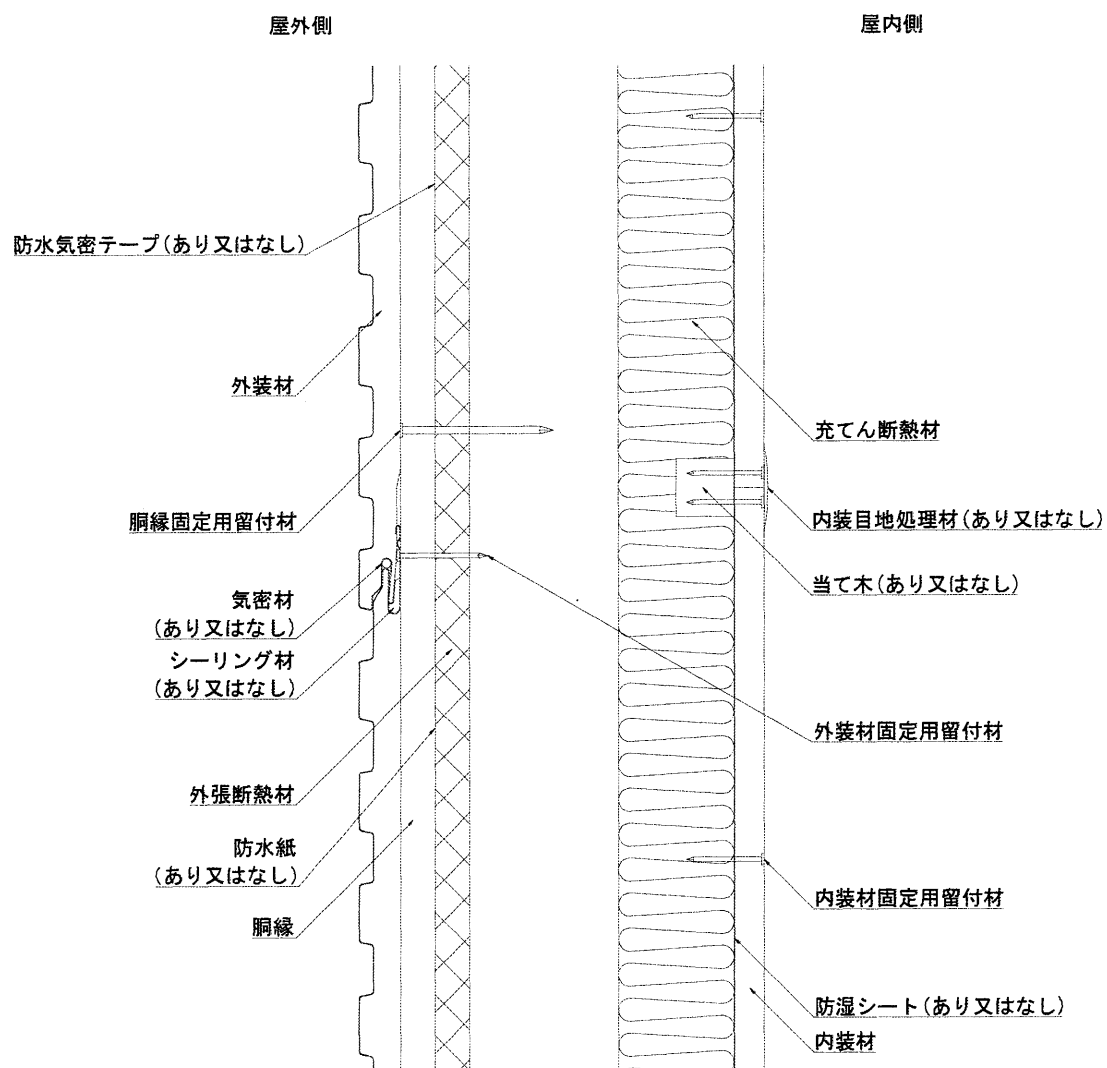
鉛直断面
