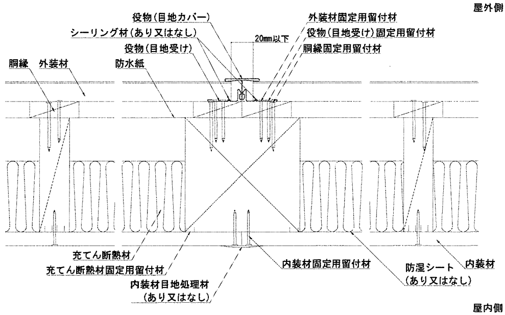
水平断面図
