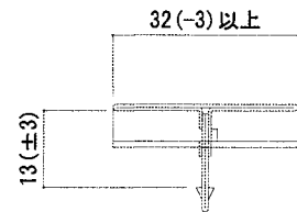
目地カバー (鋼板製) 2ピースタイプ
