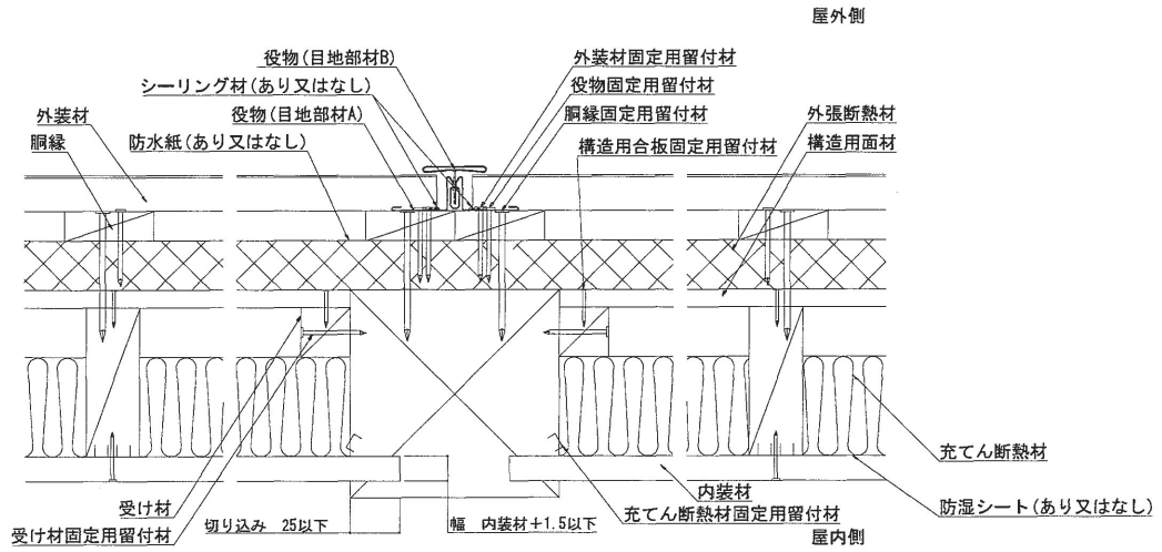
<水平断面図 面材：真壁、内装材：真壁-受け材>
