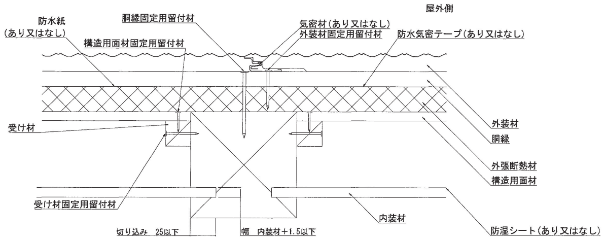
<水平断面図 面材：真壁、内装材：真壁-切り込み>
