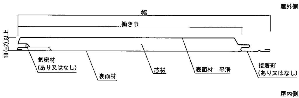
外装材断面
