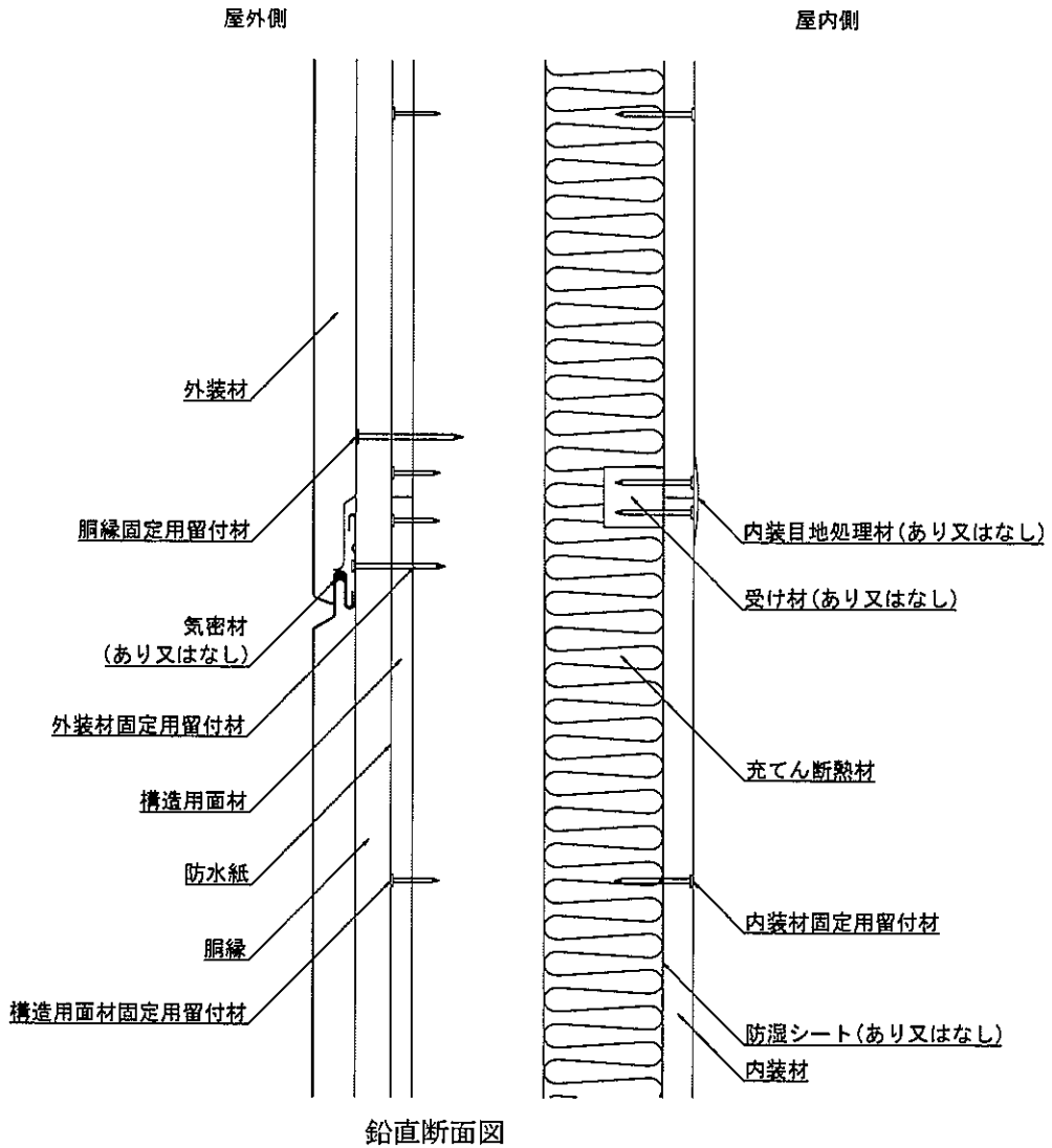
図2 構造説明図
