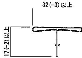
目地カバー(鋼板製)
