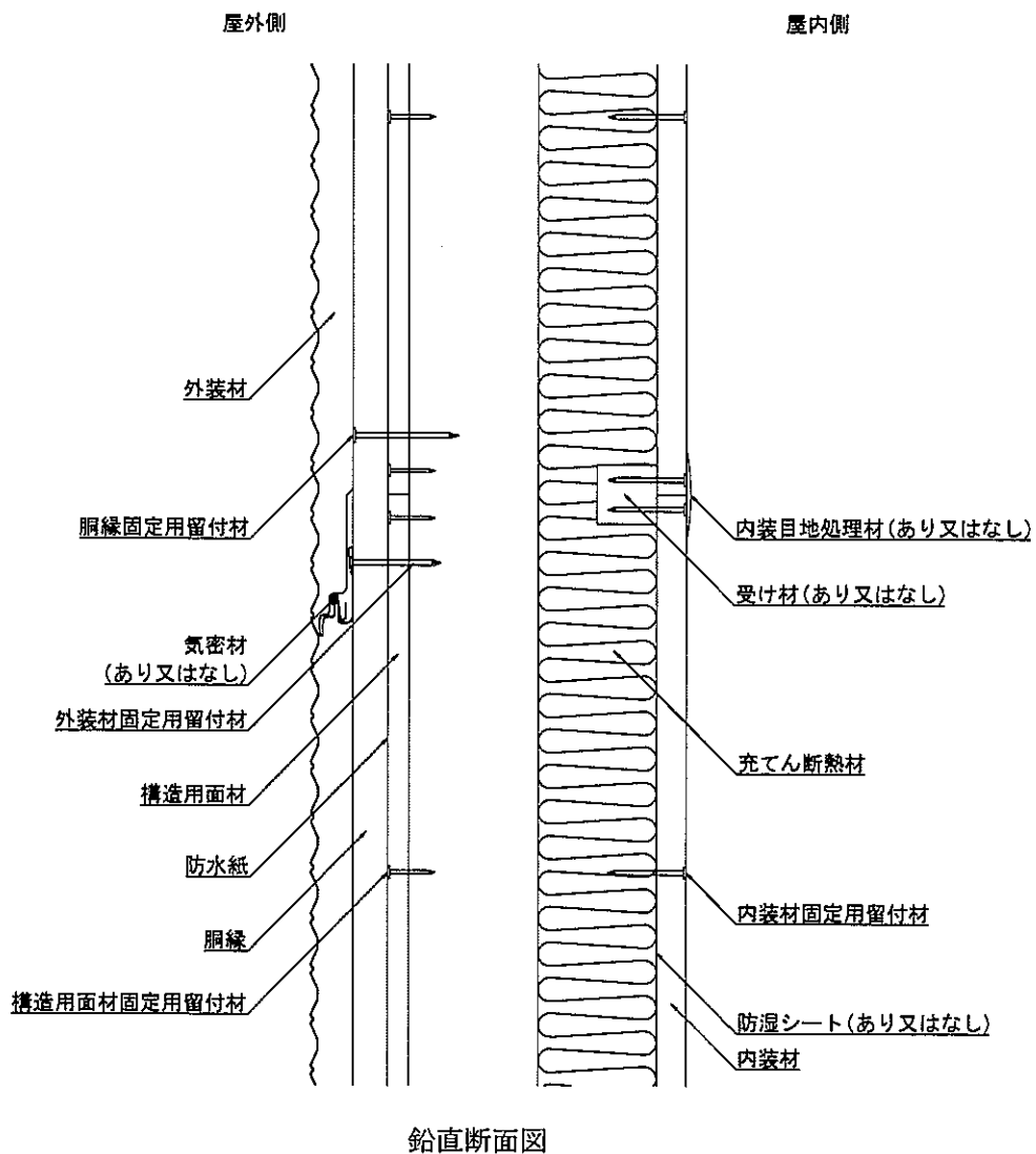
構造用面材あり 図2 構造説明図
