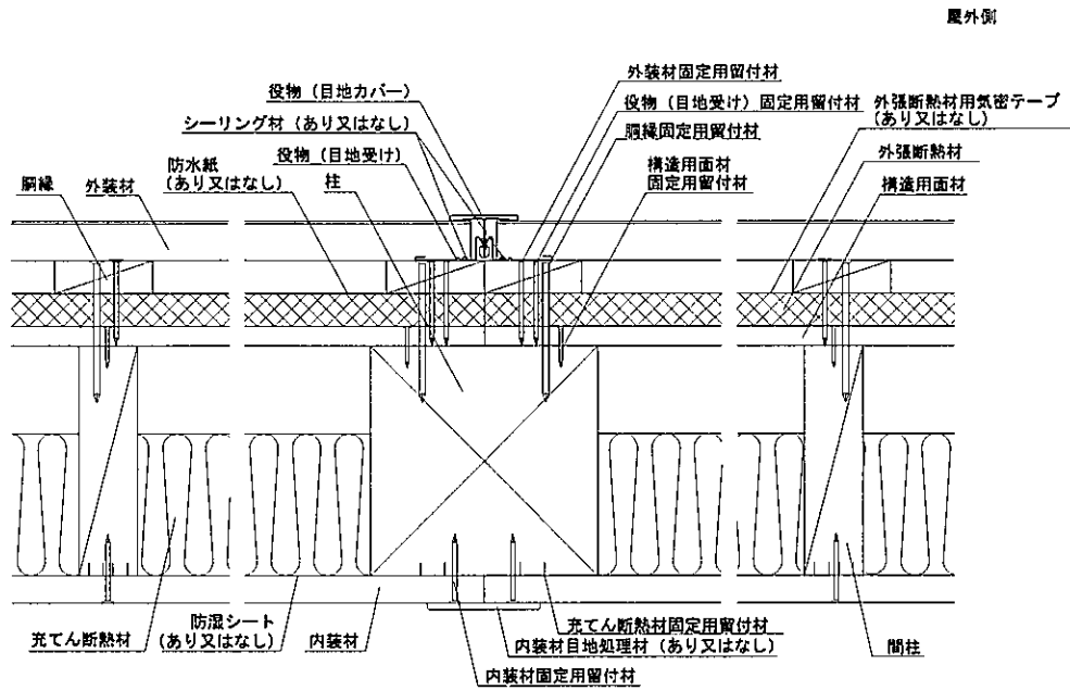
水平断面図
