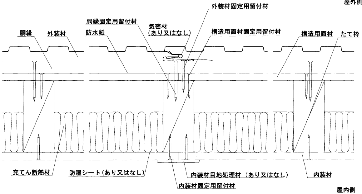
水平断面図
