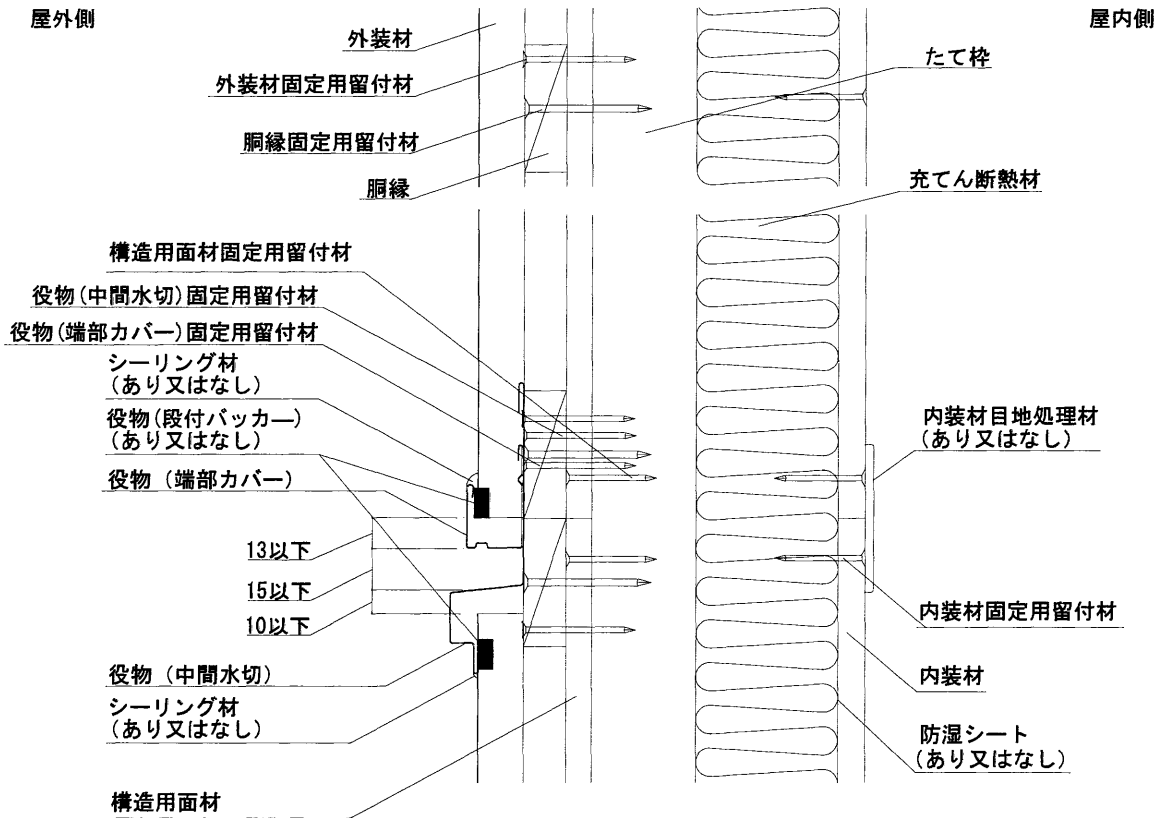
鉛直断面図
