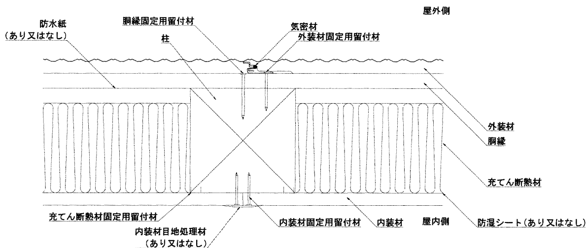
水平断面図
