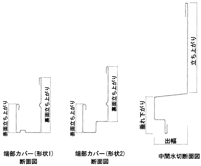
役物形状図
