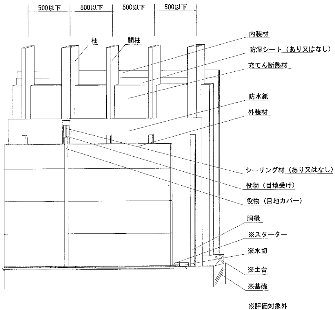
透視図
