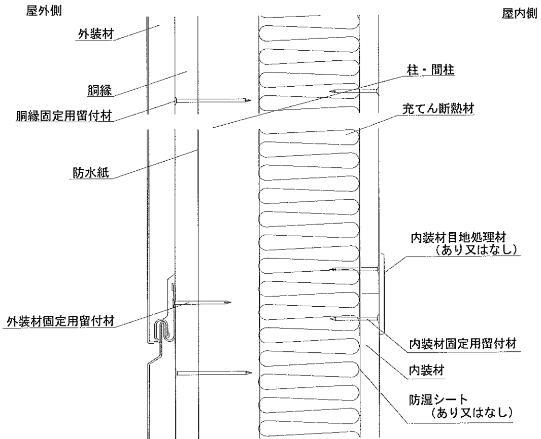
鉛直断面図
