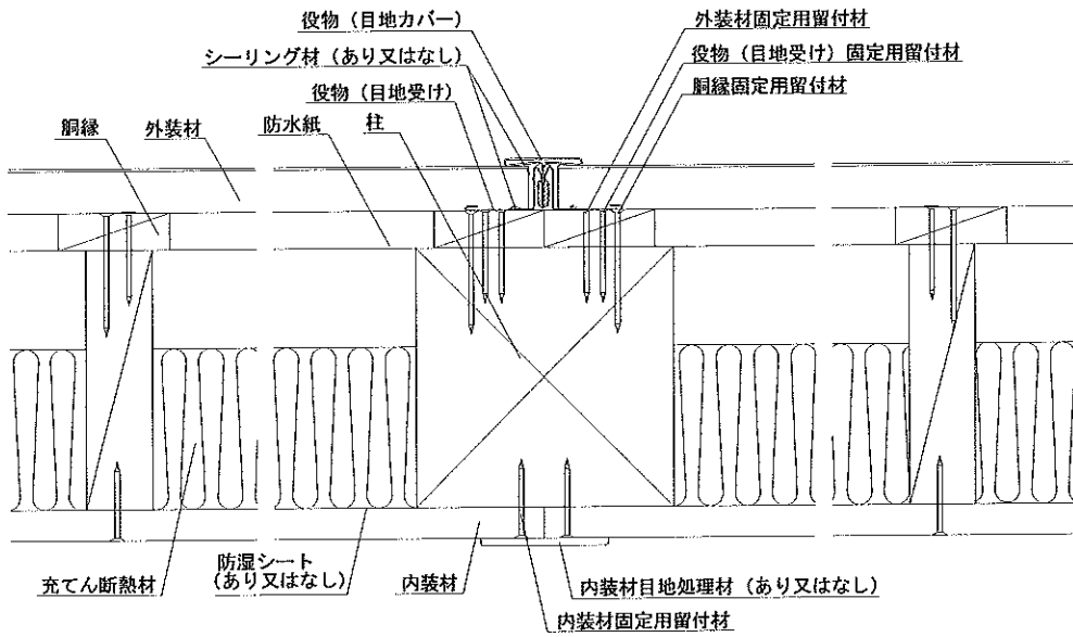
水平断面図
