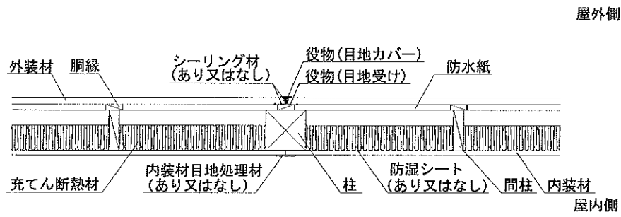
水平断面図
