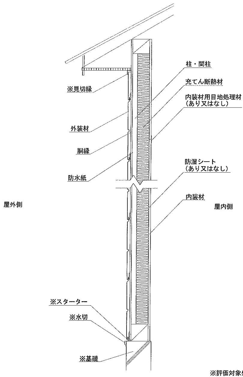
鉛直断面図 図4 施工図
