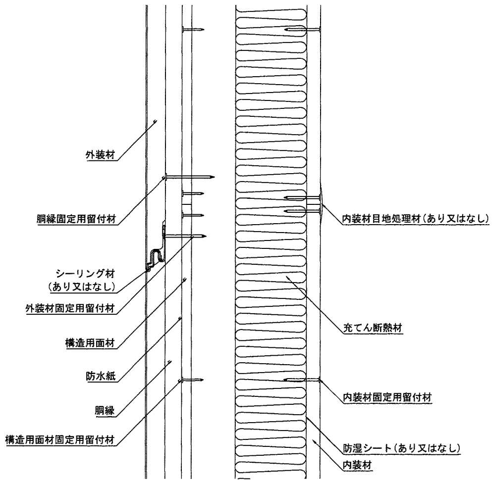
鉛直断面図
