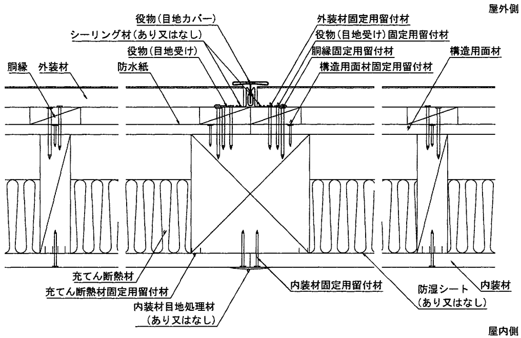
屋外側 水平断面図 屋内側
