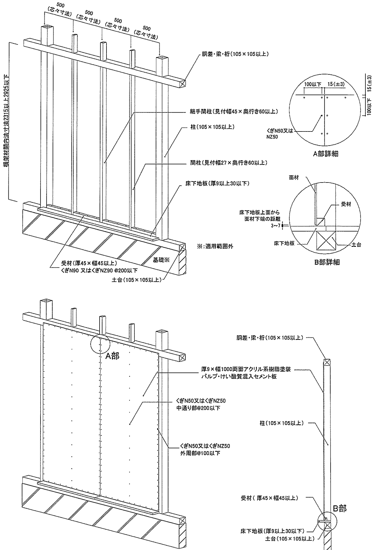
図2 施工図詳細(mm)
